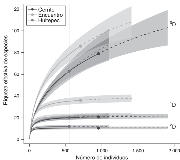
Figura 1. Curvas de interpolación (rarefacción)/extrapolación de la diversidad de heterópteros en 3 bosques secundarios de Chiapas, México, con base en los números de Hill: ^0D : riqueza (número efectivo de especies), ^1D : exponente de la diversidad Shannon, ^2D : inverso del índice de diversidad de Simpson. La línea vertical es referencia de D con respecto al sitio con el menor número de individuos (Huitepec).
