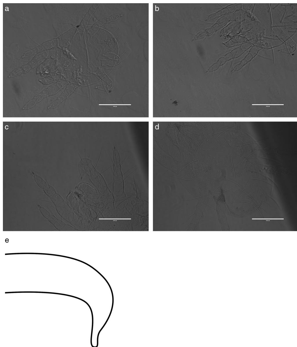
Figura 2. Aspecto general de la hembra de O. coffeae . a, Patas terminando en uña; b, setas dúplex sobre el tarso I próximas y peritrema recto; c, placa anal con 2 pares de setas anales y un par paraanales; d, eedeago curvado ventralmente y reducido abruptamente a una punta delgada (e).
